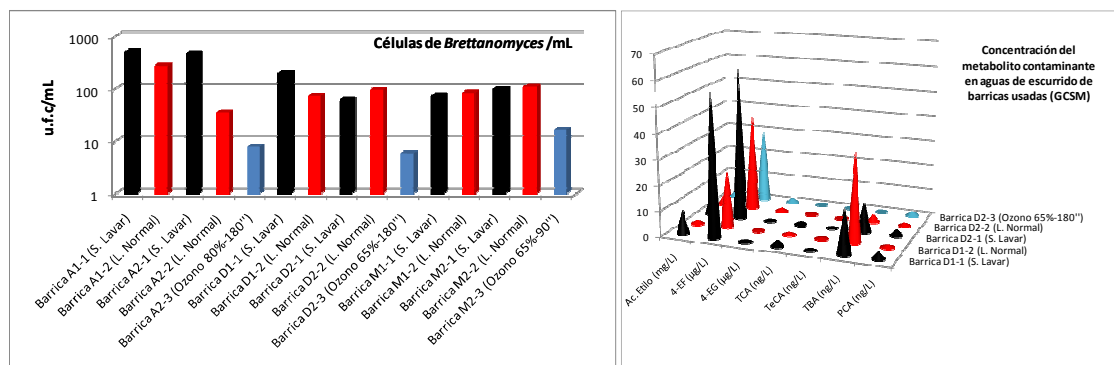
Figura 3: resultados del análisis microbiológico mediante medios de cultivo selectivos de Brettanomyces partiendo de aguas de lavado de los 3 lotes de barricas (A, D y M), gráfico izquierda y análisis mediante cromatografía de gases de metabolitos contaminantes, gráfico de la derecha.
