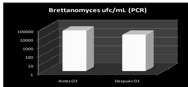
Figura 8: resultados del análisis microbiológico de Brettanomyces en aguas de lavado mediante PCR a tiempo real.
