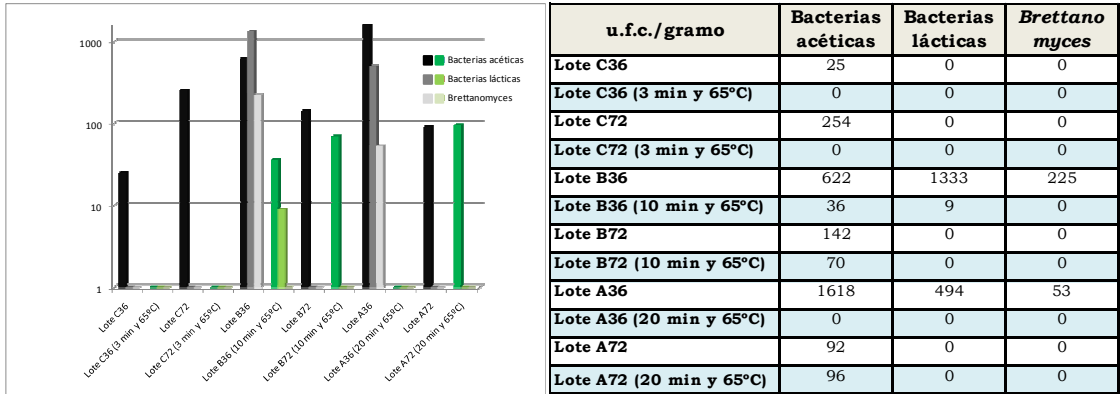
Figura 11 y Tabla 5: resultados del análisis microbiológico de 5 barricas homogéneas. Figura 11: en negro y gris antes del tratamiento, en verde después del tratamiento. Tabla 5: filas con fondo blanco antes del tratamiento y filas con fondo oscuro después del tratamiento con microondas.
